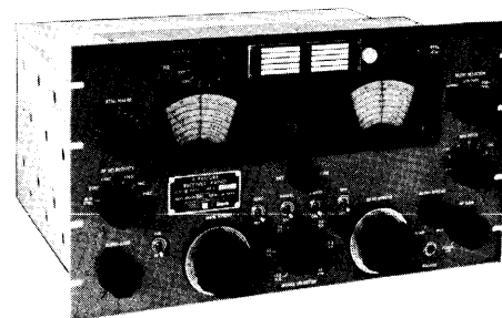
GPR-90-RX, GPR-90RXD OCDM Item No. R-02, R-16
