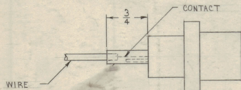
WIRING DETAIL ITEM 20 (MS 3102 A32-7P)
