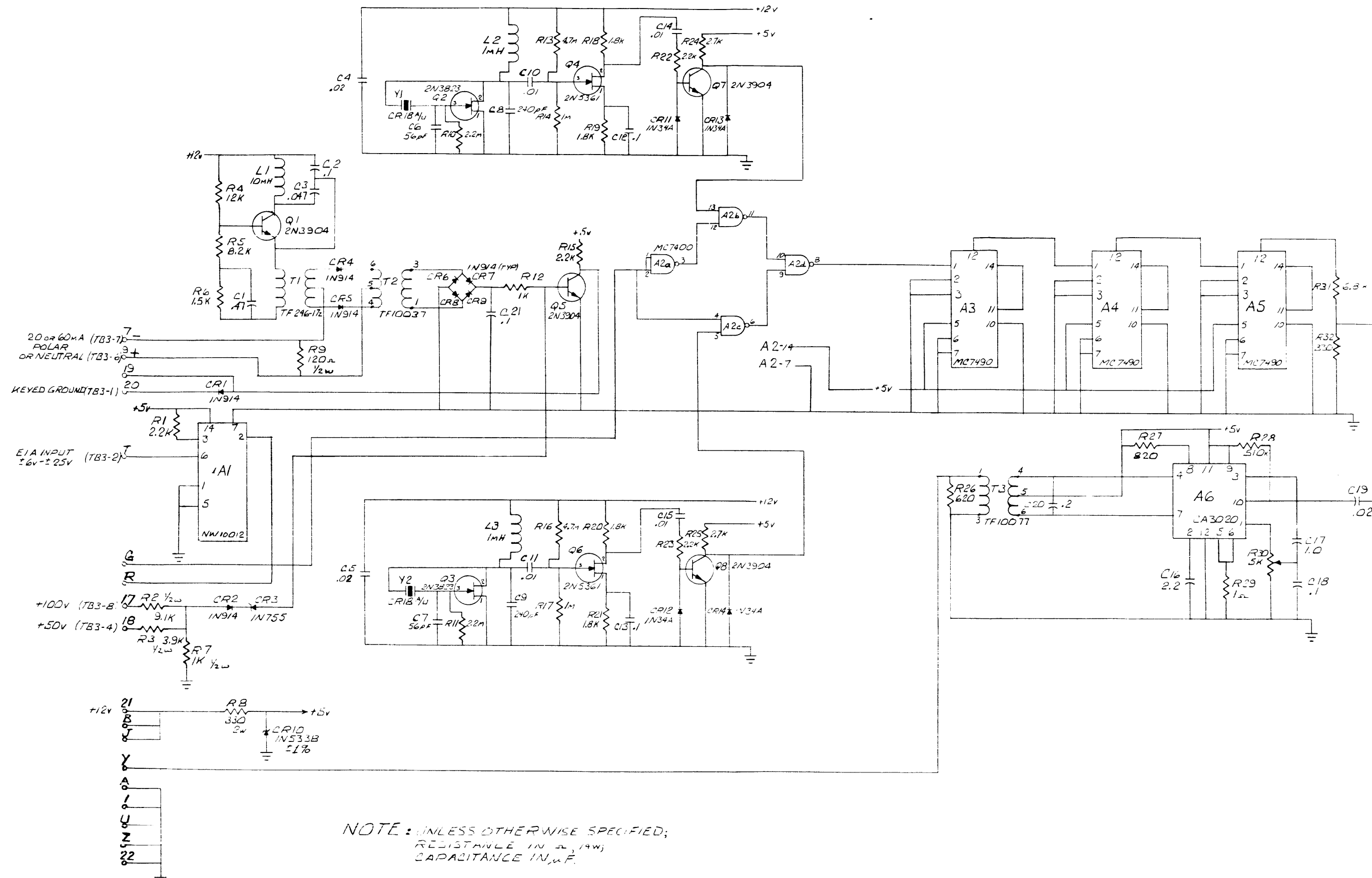
A1 FREQUENCY SHIFT FIG. 7-12
